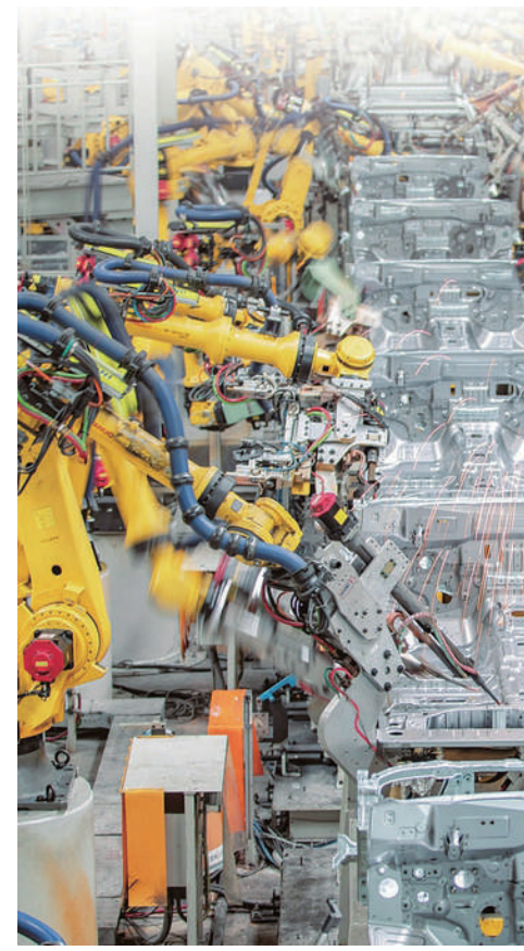
3月1日,在长城汽车重庆永川生产基地焊装车间,智能化焊接机器人在进行焊接作业。
