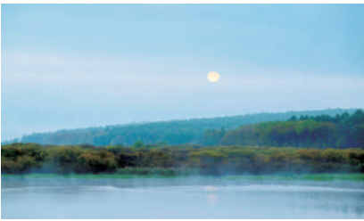
这是9月27日凌晨在黑龙江市拜泉县拍摄的月亮。今年农历八月上演“十五的月亮十七圆”，最圆时刻出现在9月27日0时49分。新华社发 姜晓峰 摄
